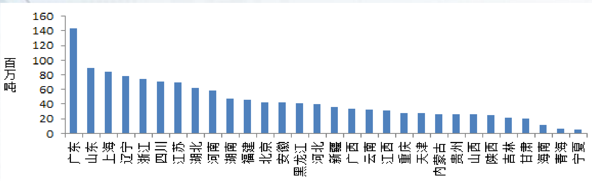
▲各省石油碳排放情况，2017年
