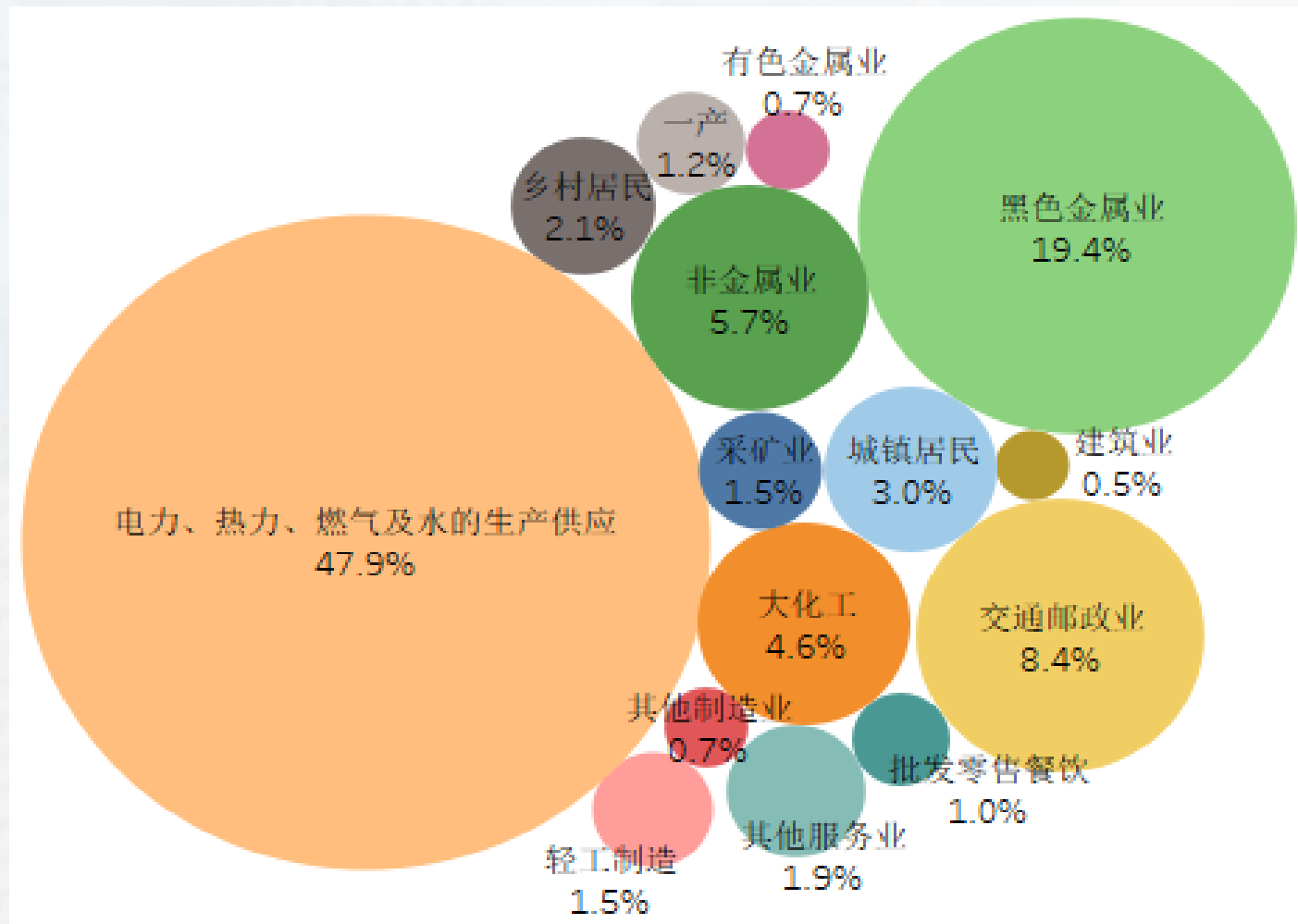
▲分部门排放情况，2017年
